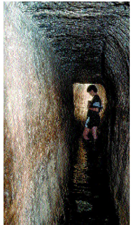
Los trabajadores del rey Ezequías lograron una tremenda hazaña de ingeniería al cavar un gran túnel (a la derecha) a través de la piedra caliza debajo de Jerusalén con el fin de proveer una fuente segura de agua a la ciudad que enfrentaba la invasión asiria. Esta inscripción describe cómo los obreros cavaron por ambos extremos hasta que llegaron a la mitad y terminaron así la monumental obra.
